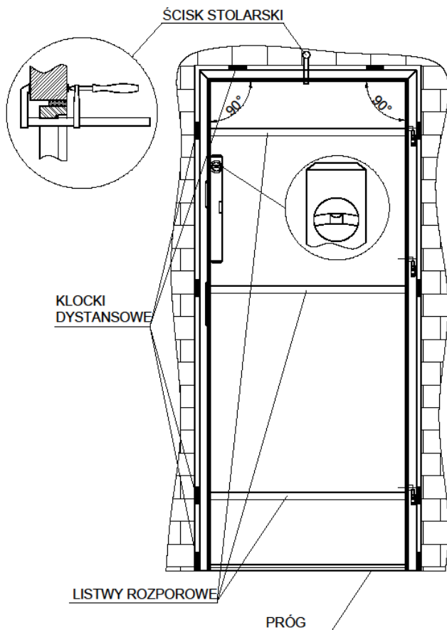
Rys. 1. Rozmieszczenie klocków dystansowych i listew rozporowych
