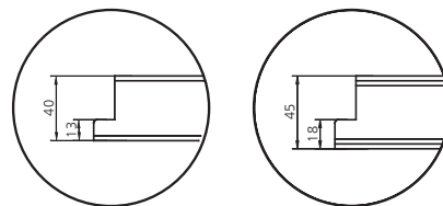
Przekrój skrzydła
