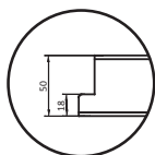
Przekrój poprzeczny skrzydła EI 230 F1, F2
