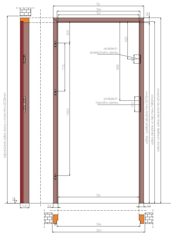
TABUĽKA ROZMEROV NÁKRES 1
